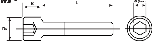
Dimensions to BS EN ISO 4762 DIN 912
